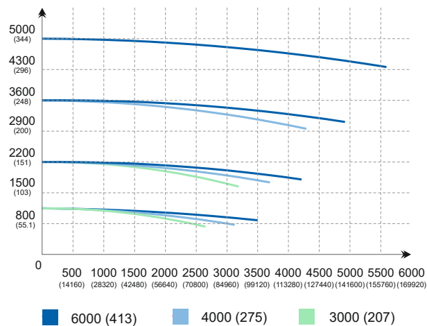
Графики расхода
