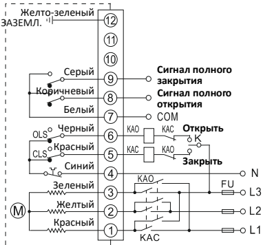
ТИП H: 3-фазная цепь управления переменного тока (с переключателем пассивного контакта)
