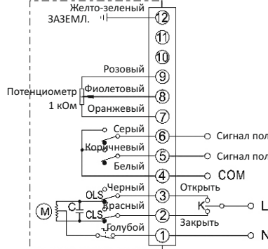
ТИП F: С датчиком положения
