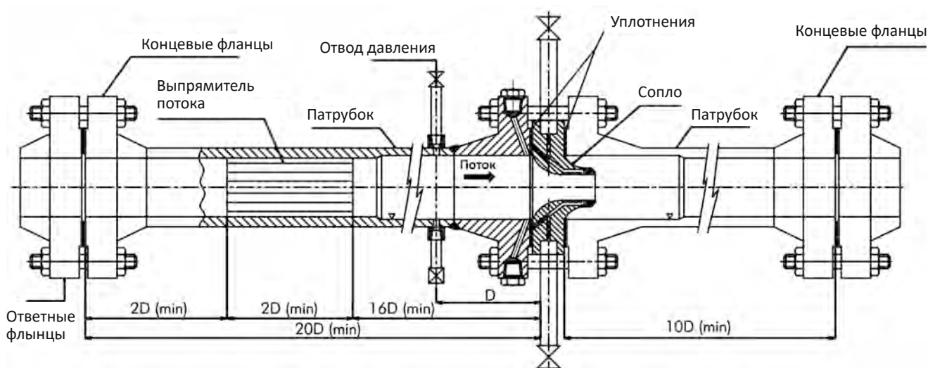
Сопло в сборе по ASME PTC-6
