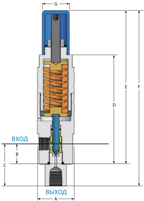
[клапан с 1 входом] Давление: 68,9 ~ 689 бар (1000 ~ 10 000 фунт/кв.дюйм)
