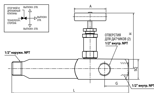
V46GRL. Удлиненный манометрический клапан
