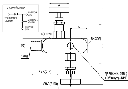
V46GRL. Удлиненный манометрический клапан
