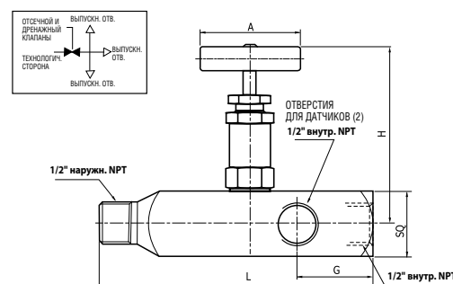
V46GR. Манометрический клапан
