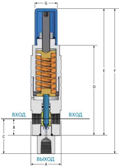
[клапан с 2 входами] Давление: 68,9 ~ 689 бар (1000 ~ 10 000 фунт/кв.дюйм)
