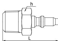
SV: шток без запора
