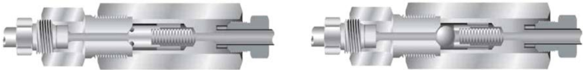
Обратный клапан с уплотнительным кольцом/шаровой
